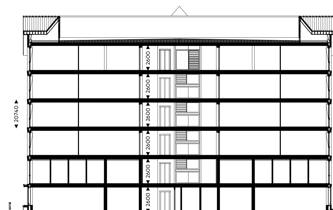
principedoorsnede
