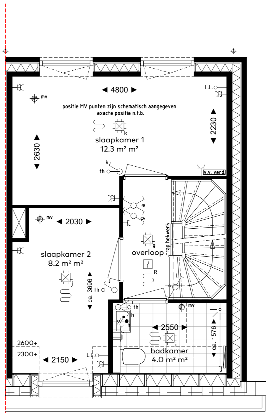
EERSTE VERDIEPING
