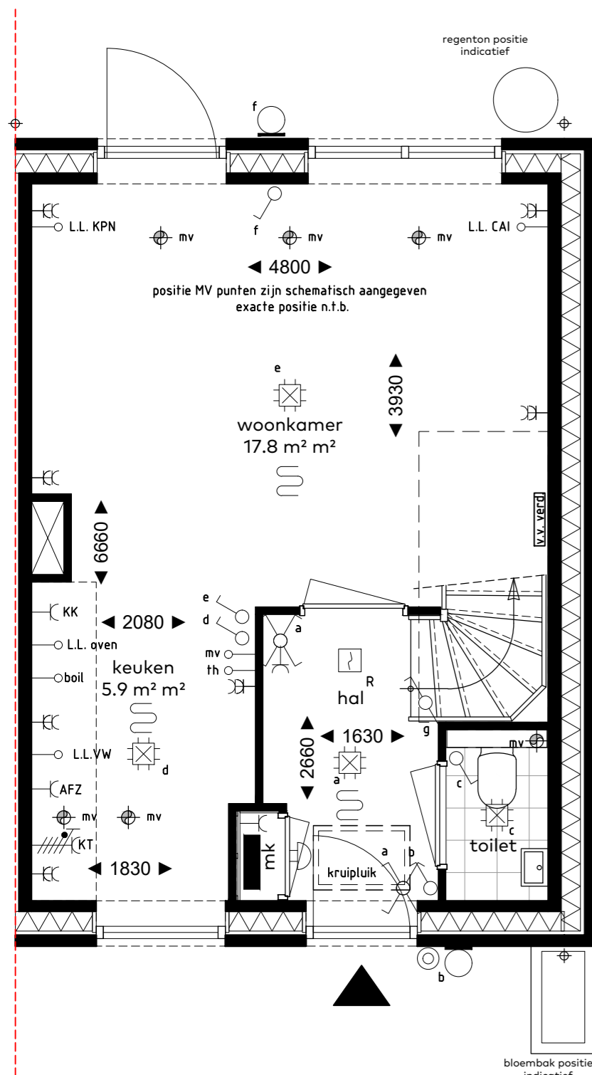
BEGANE GROND
