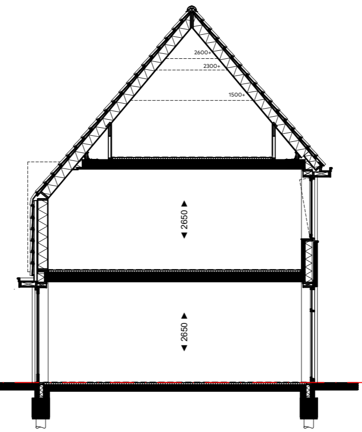
PRINCIPEDOORSNEDE C-C schaal 1:100
