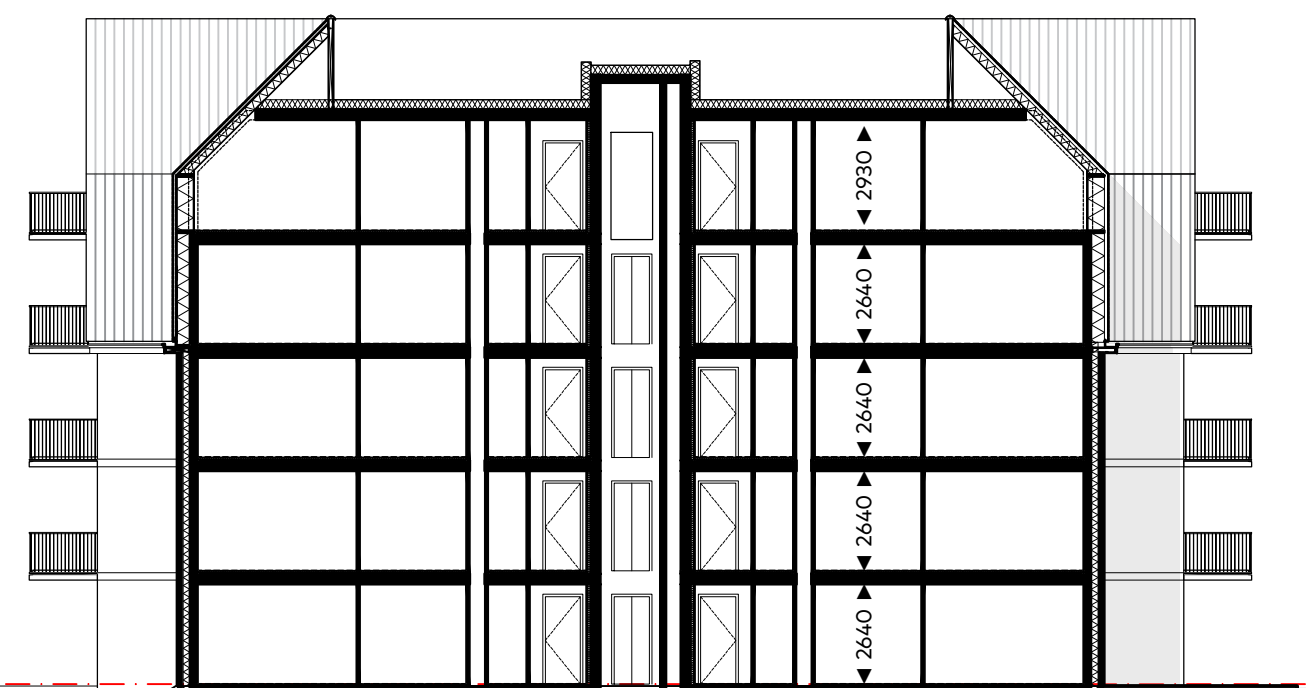
PRINCIPE DOORSNEDE
