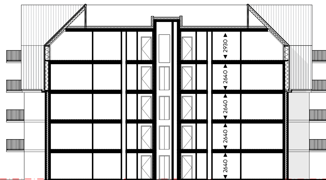
PRINCIPE DOORSNEDE
