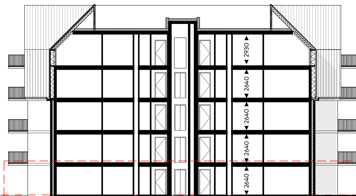
PRINCIPE DOORSNEDE
