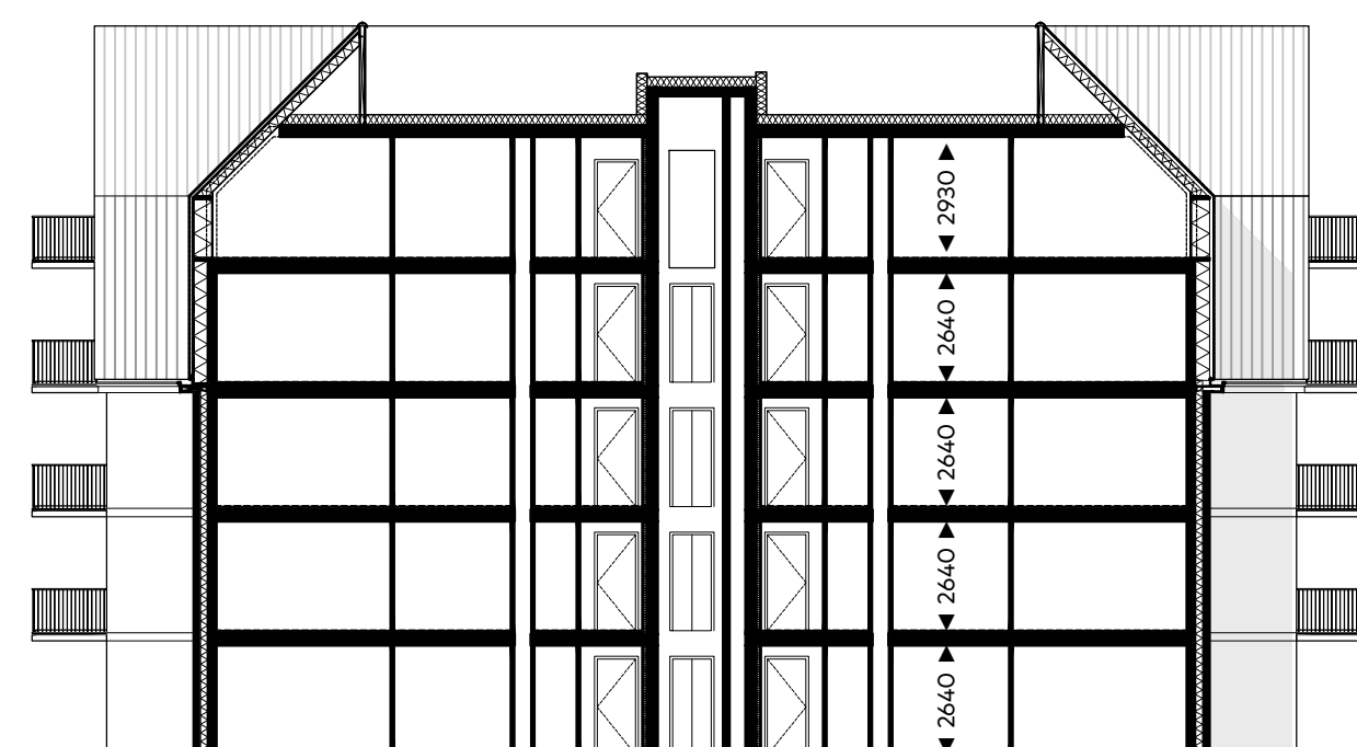
PRINCIPE DOORSNEDE
