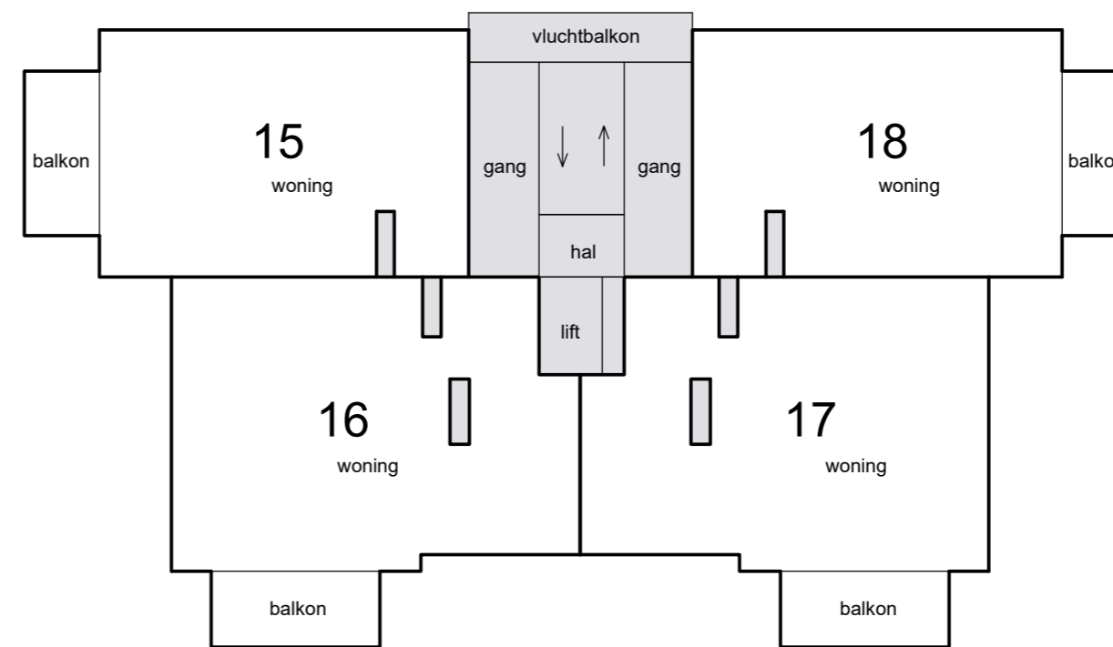
4e verdieping
