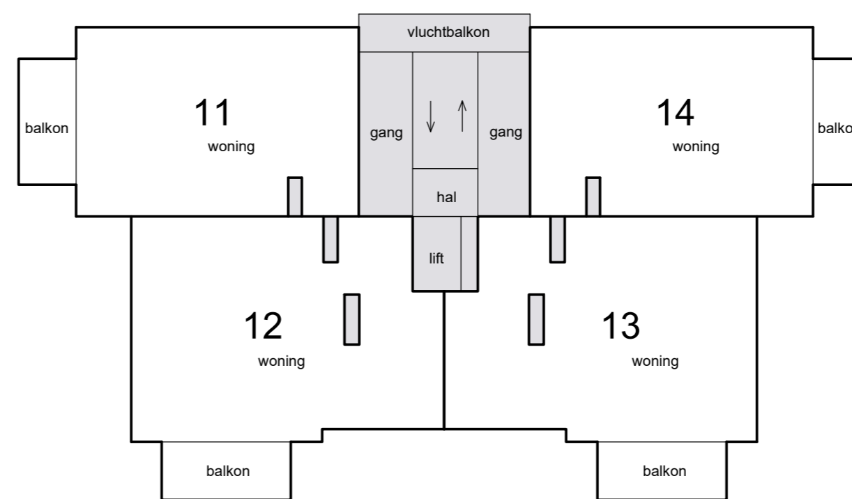
3e verdieping
