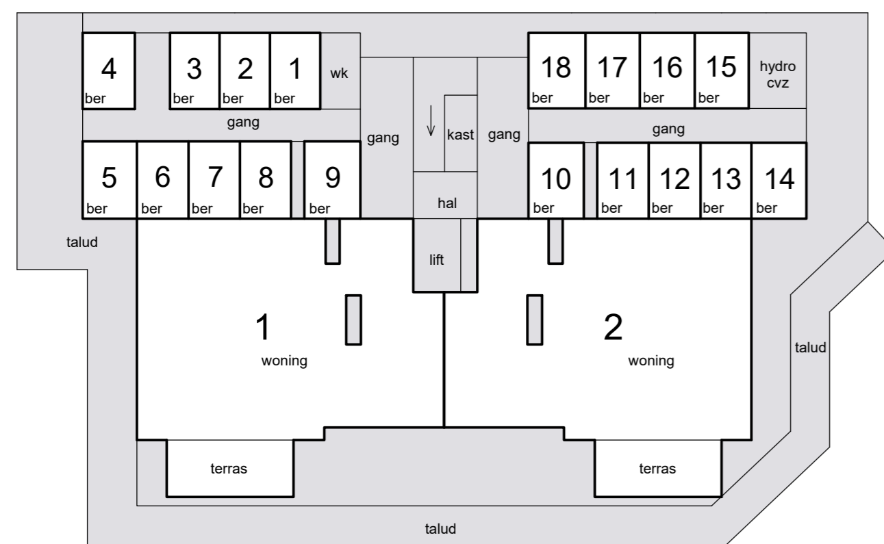
begane grond
